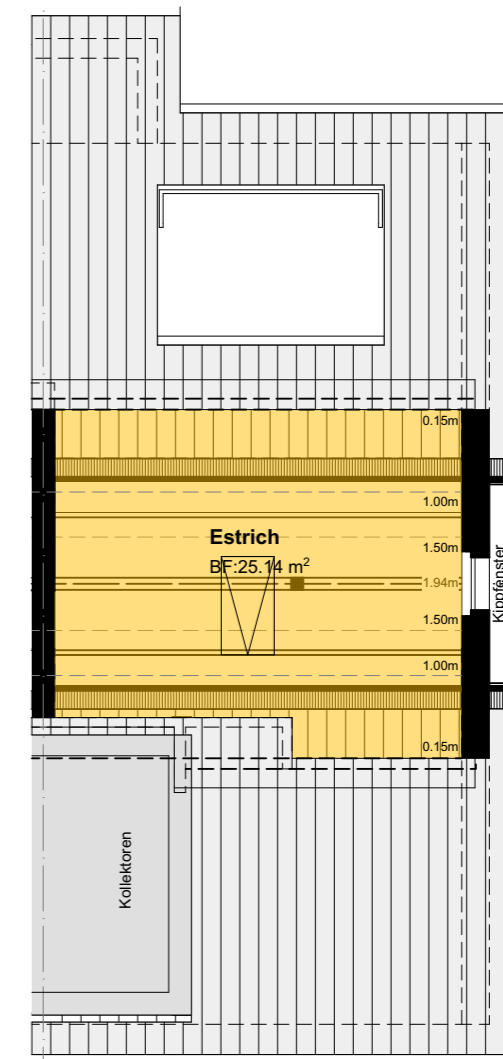
Estrichgeschoss
