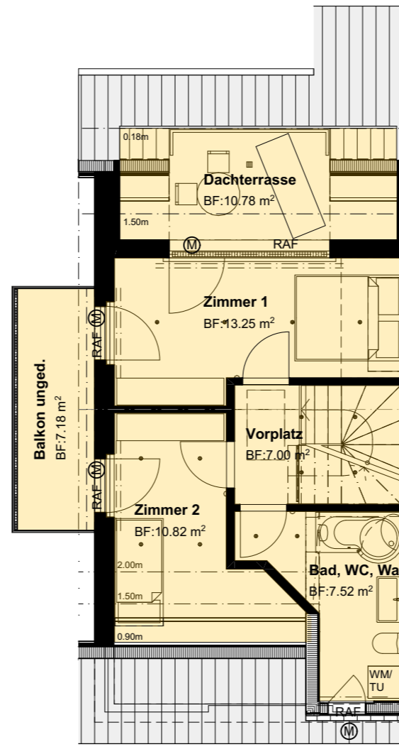
Dachgeschoss
