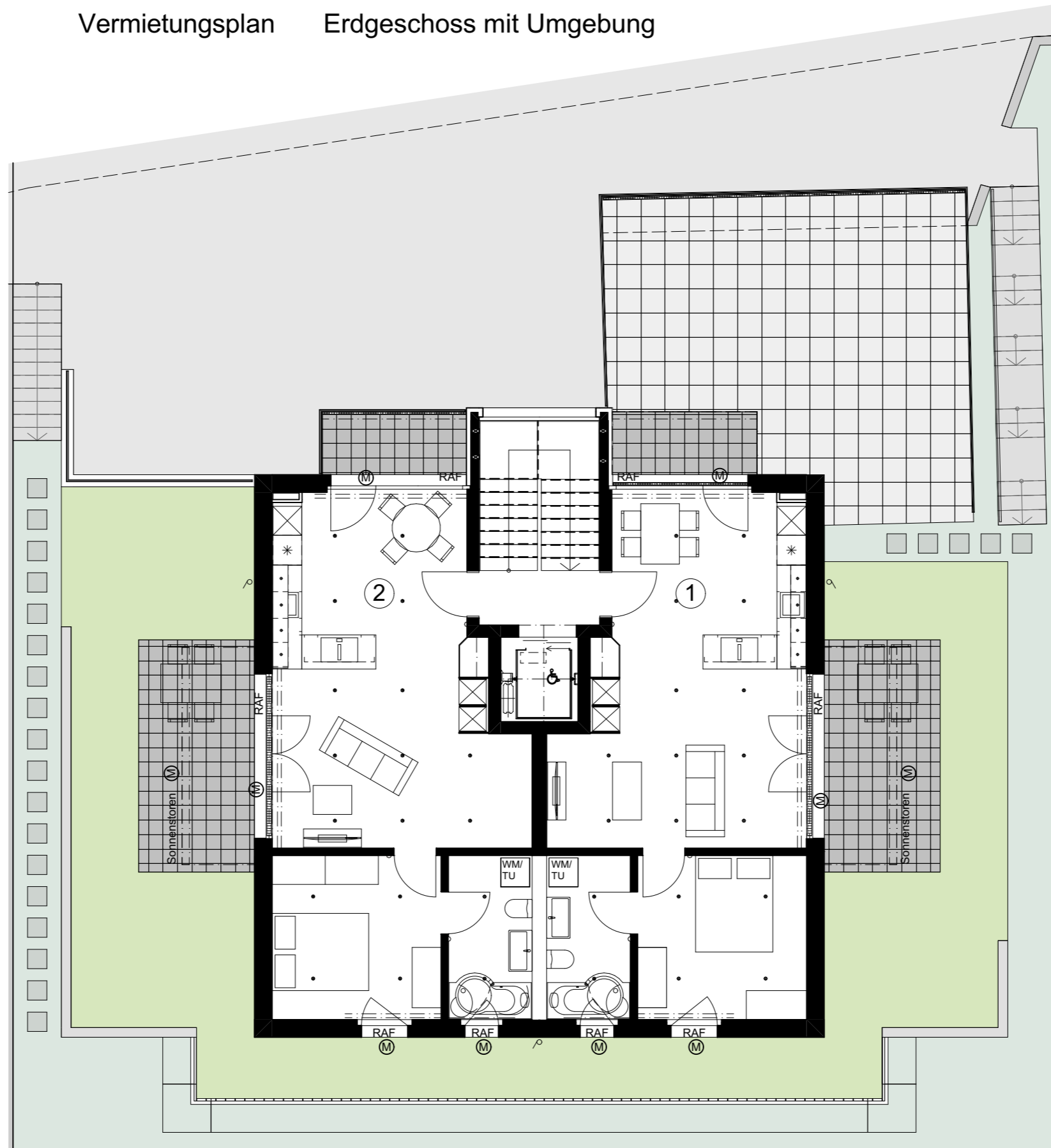
Erdgeschoss mit Umgebung
