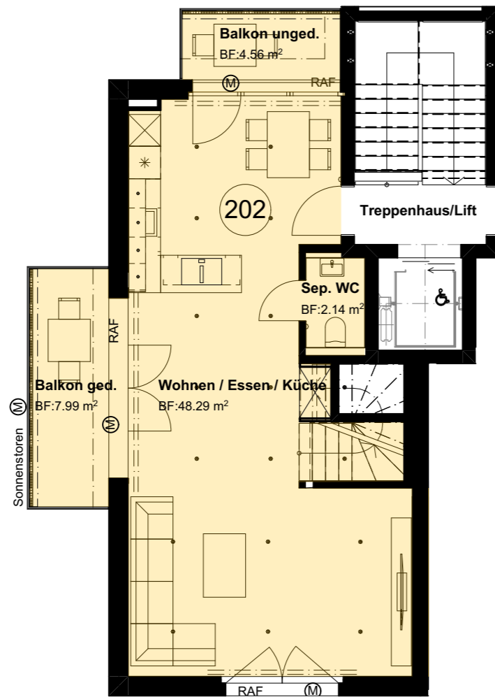
2.Obergeschoss
